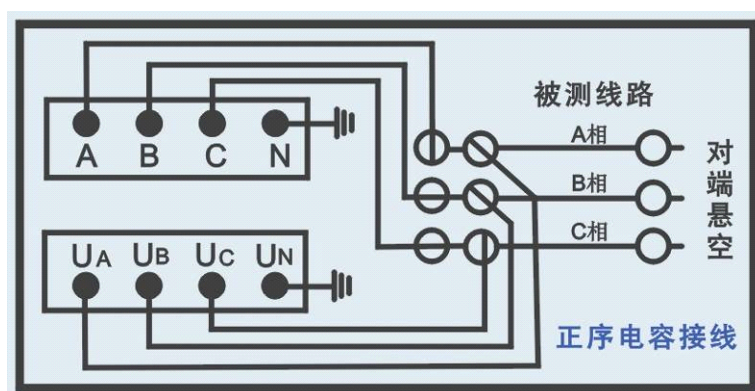
图 5—4、正序电容接线
