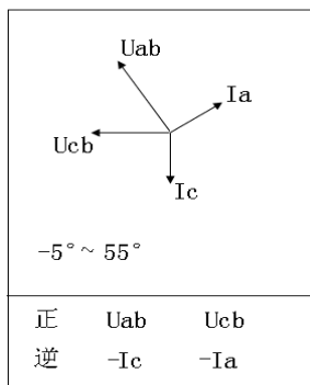
A、C相电流相间接错并接反
