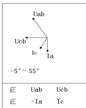
A、B、C三相电压接线正确
