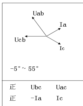
A、B、C三相电压分别接C、A、B
